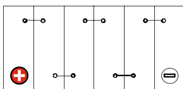
Schaltung 1
