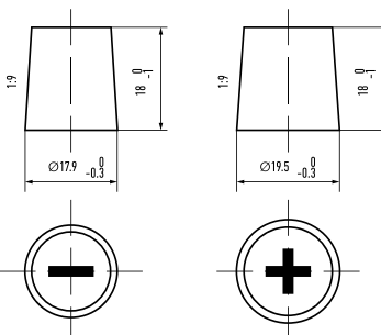
Anschlusspole 1
