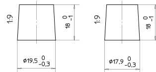
Anschlusspole 1
