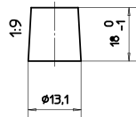
Anschlusspole 3
