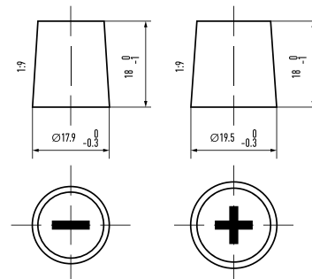
Anschlusspole 1
