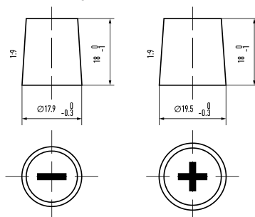
Anschlusspole 1
