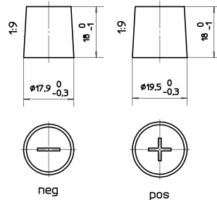
Anschlusspole 1
