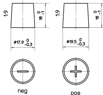
Anschlusspole 1
