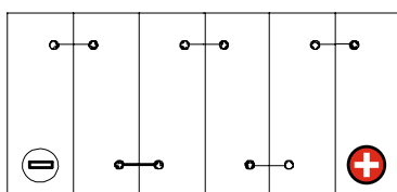
Schaltung 0
