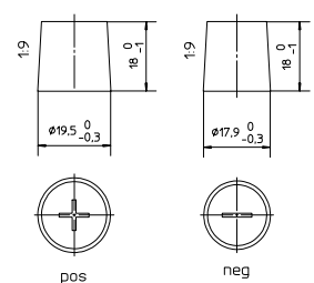
Anschlusspole 1
