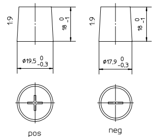
Anschlusspole 1
