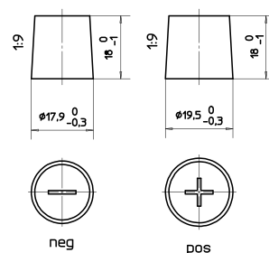
Anschlusspole 1
