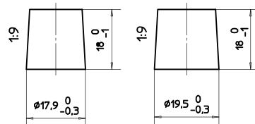
Anschlusspole 1
