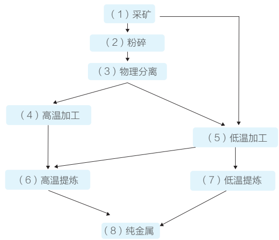
附图 2. 金属开采冶炼流程图 [47]
