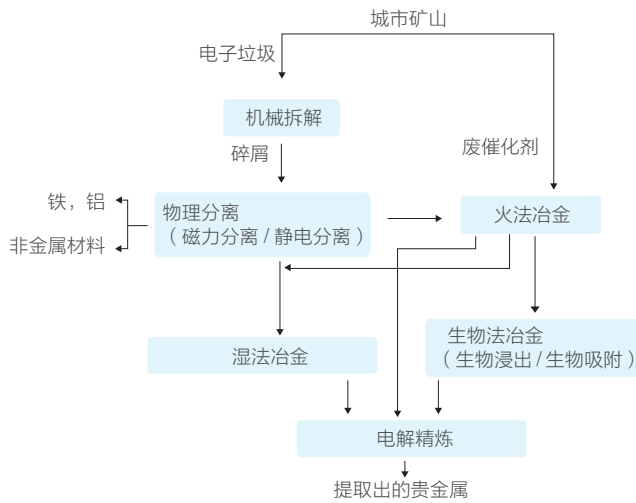
附图 1. 从废旧电子产品中冶炼稀贵金属的流程 [46]
