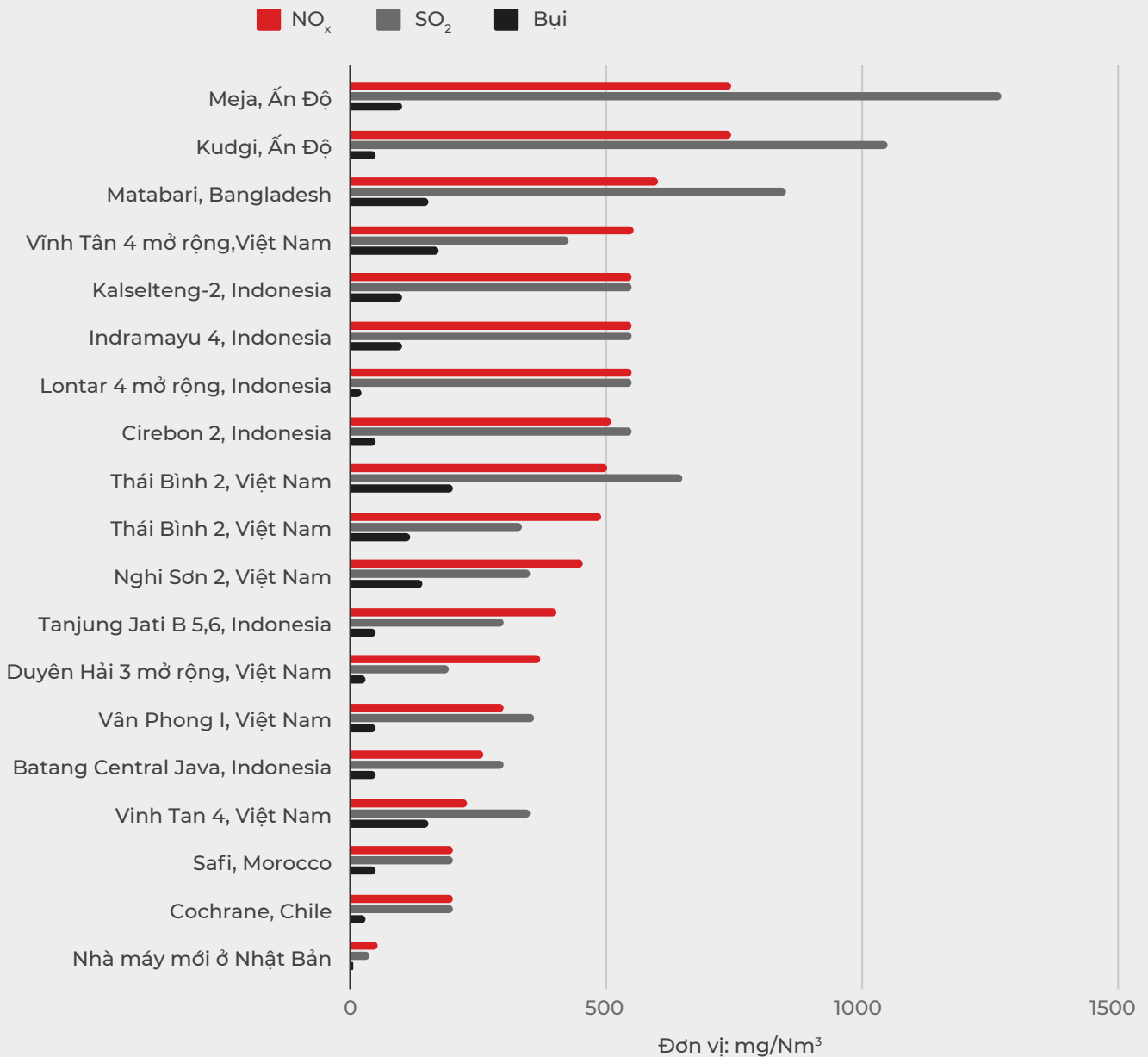
Hình: Giới hạn phát thải đối với các chất ô nhiễm không khí NO x , SO 2 và bụi của các nhà máy điện than ở Nhật Bản 6 so với các nhà máy điện than do Nhật Bản đầu tư ở nước ngoài.
