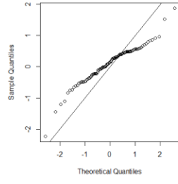
E Normal Q-Q Plot
