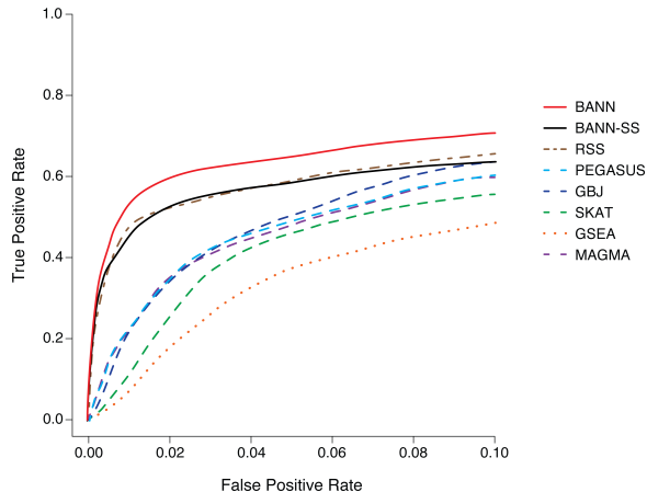
(D) SNP-Set Methods (Polygenic Traits)
