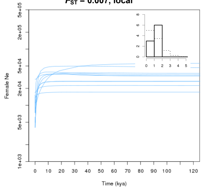
F_{ST} = 0.007 , local
