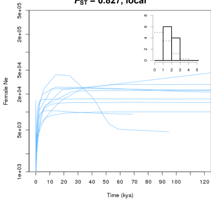
F_{ST} = 0.827 , local
