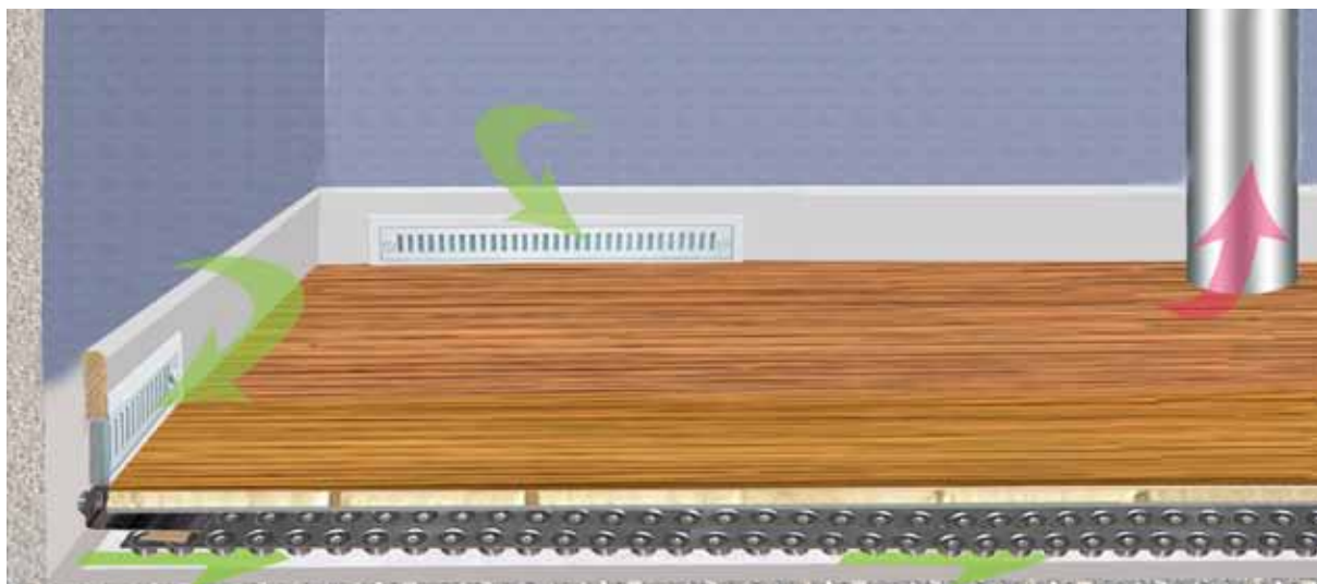
Principskiss av Optiventsystemet
