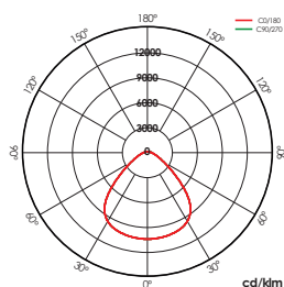
150W 90°
