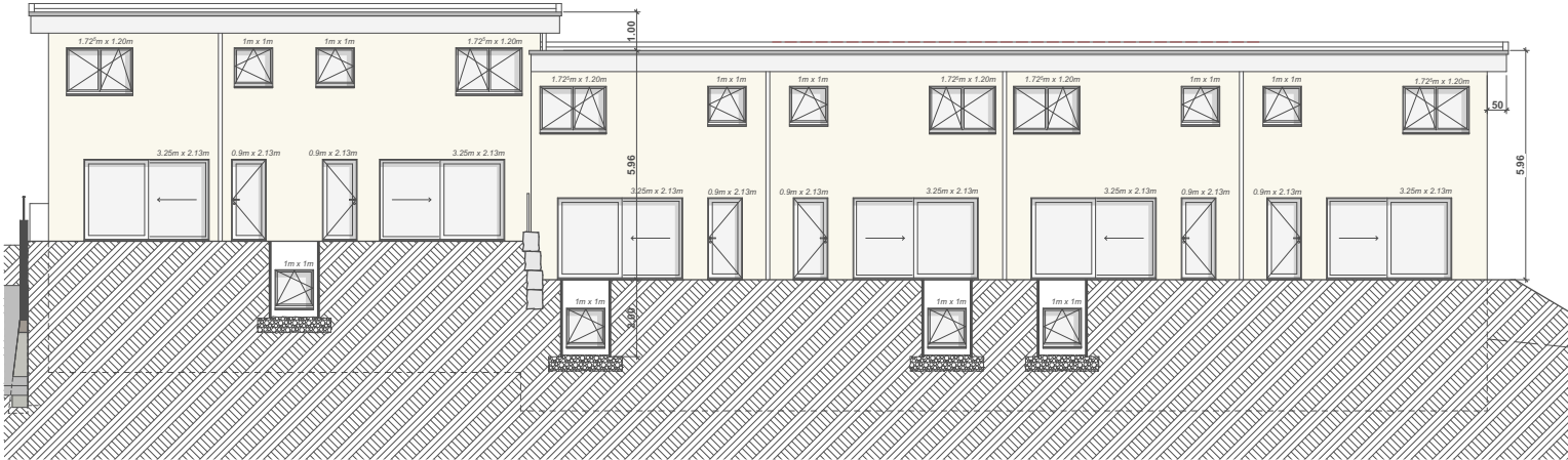
Ansicht Ost
