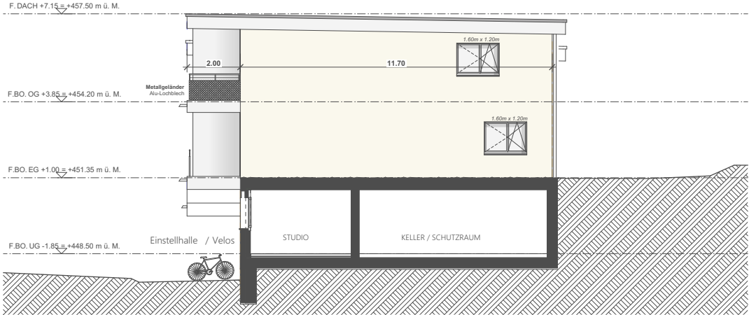
Ansicht Süd
