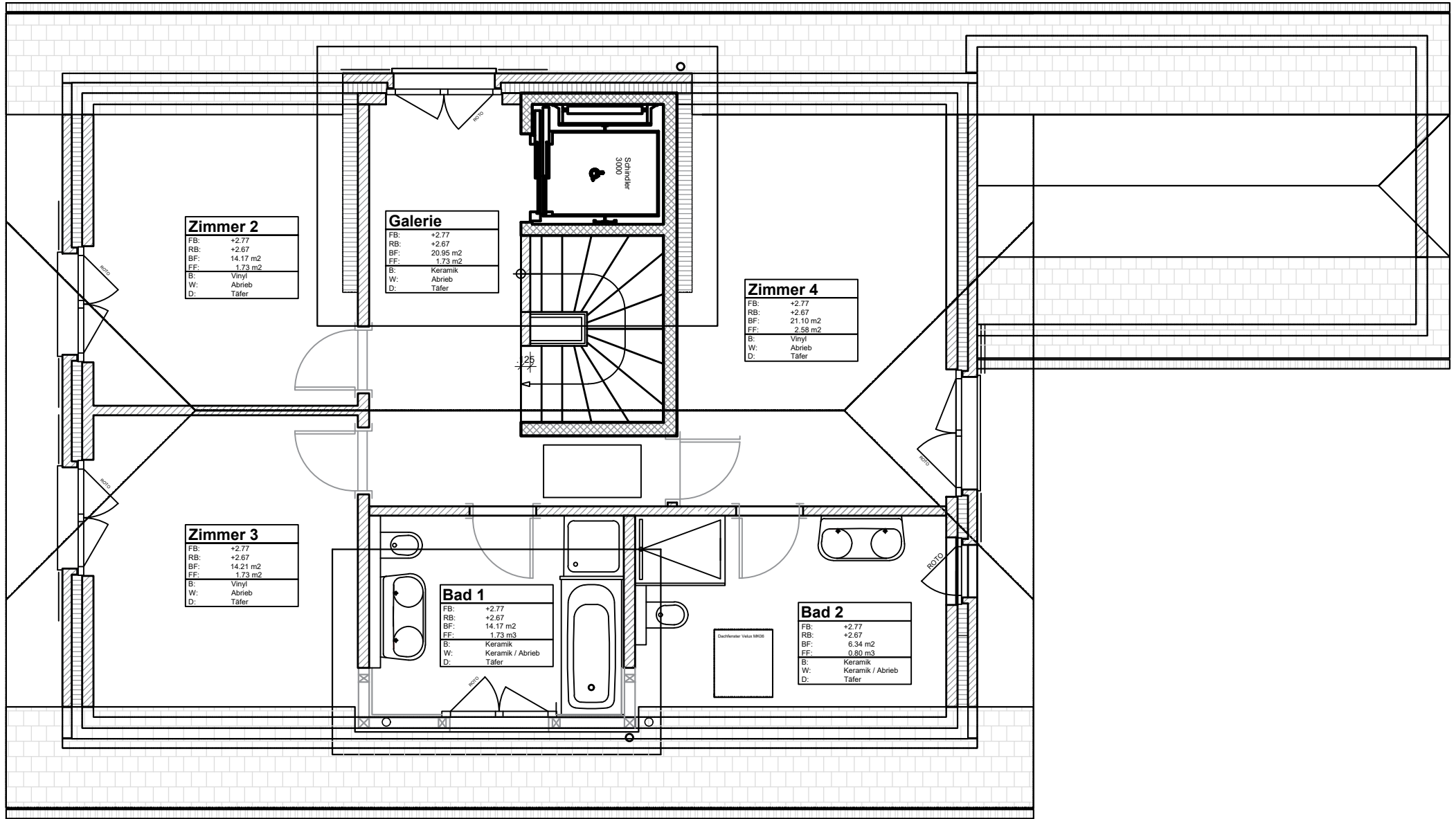
Obergeschoss
