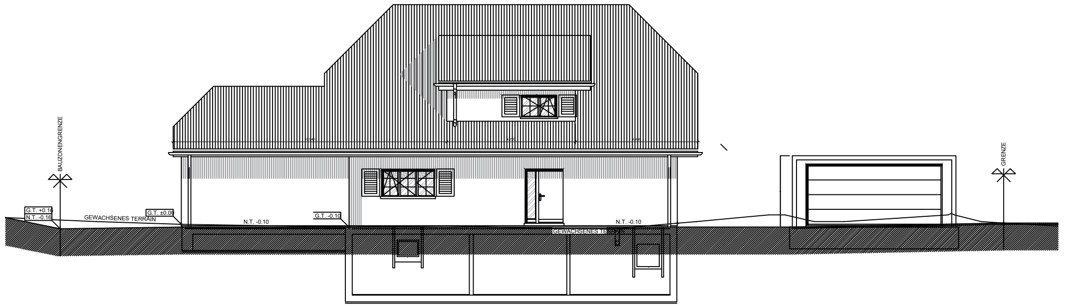
NORD-OST FASSADE
