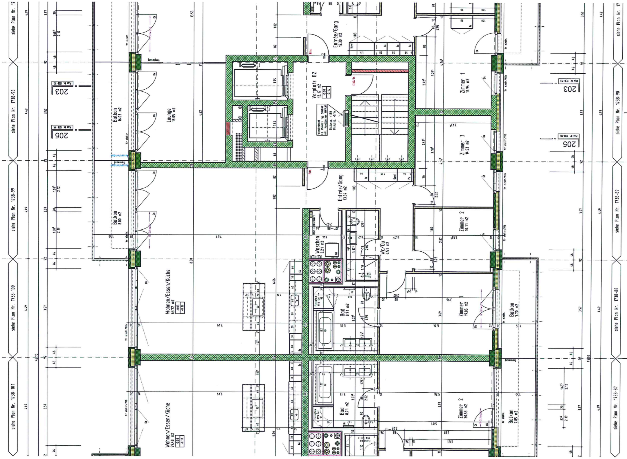
Wohnung B2.071 143.68 m 2
