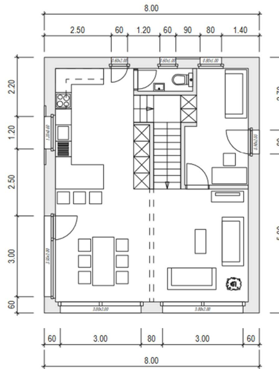
Grundriss EG
