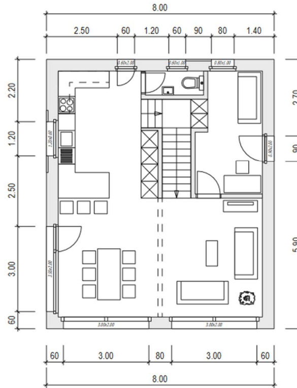
Grundriss EG
