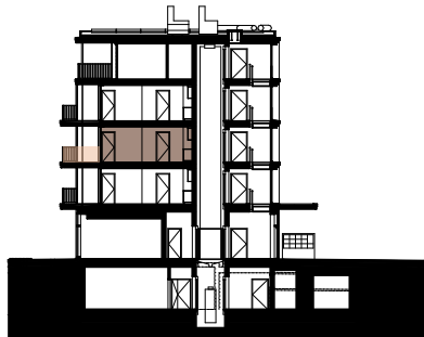
Übersichtsplan Querschnitt
