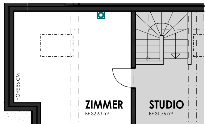
DACHGESCHOSS
