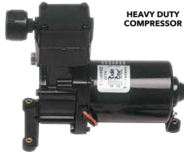
ULTRR9335 12 VOLT. • 145 PSI. • 1/8" NPT
