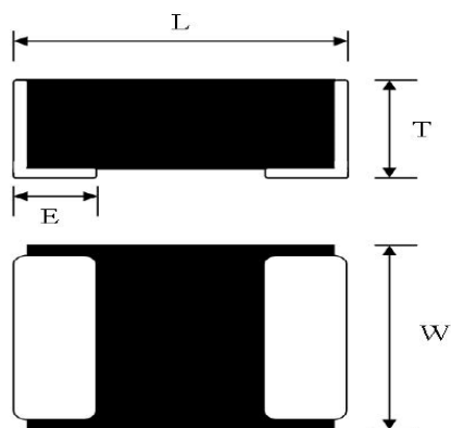
201610~252012 系列尺寸圖
