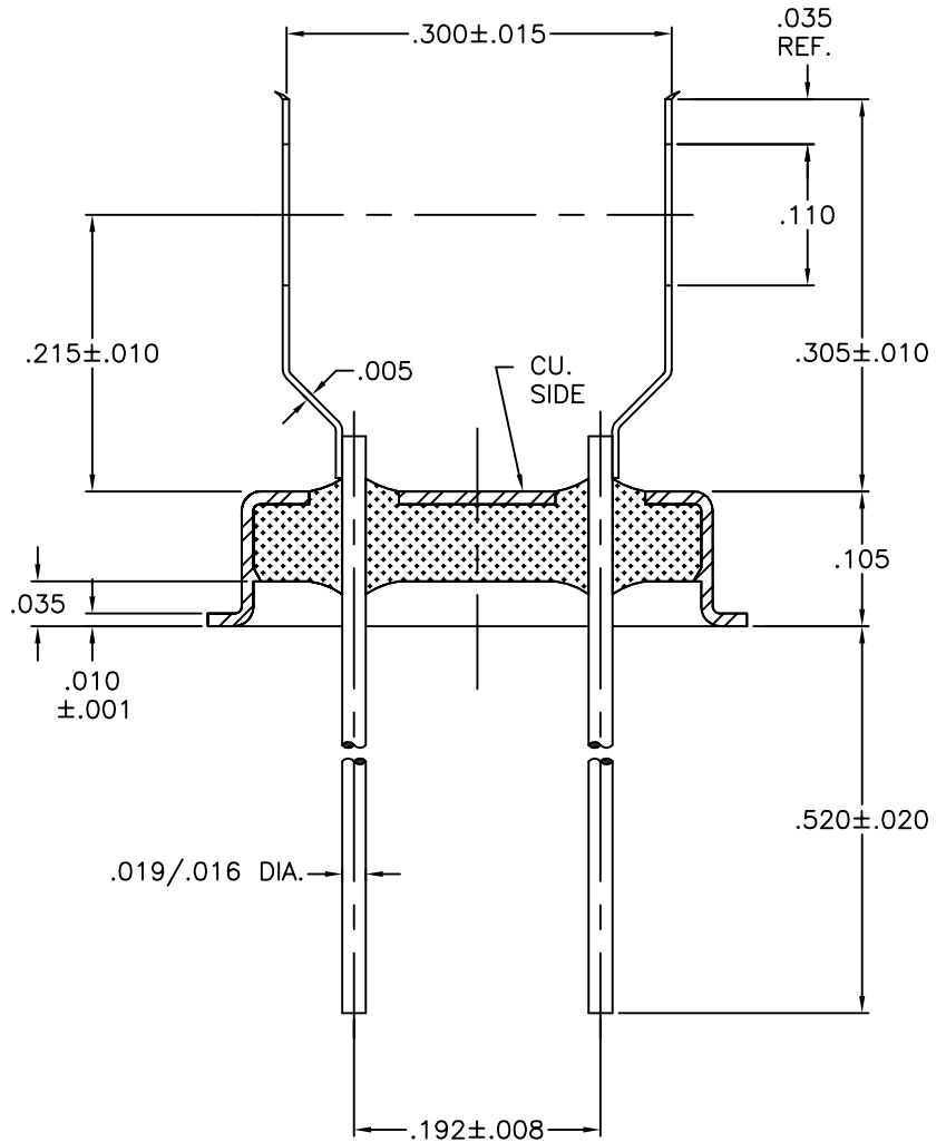
SECTION A-A
