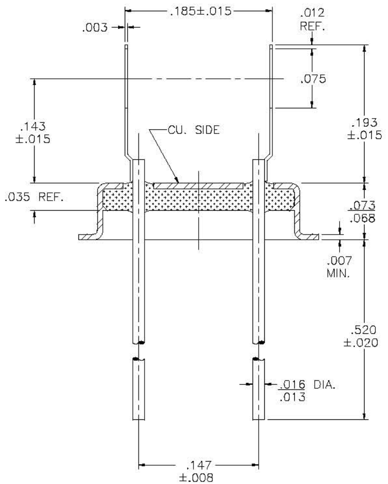
SECTION A-A
