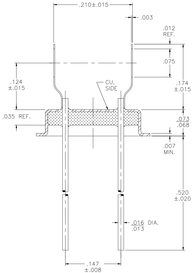
SECTION A-A
