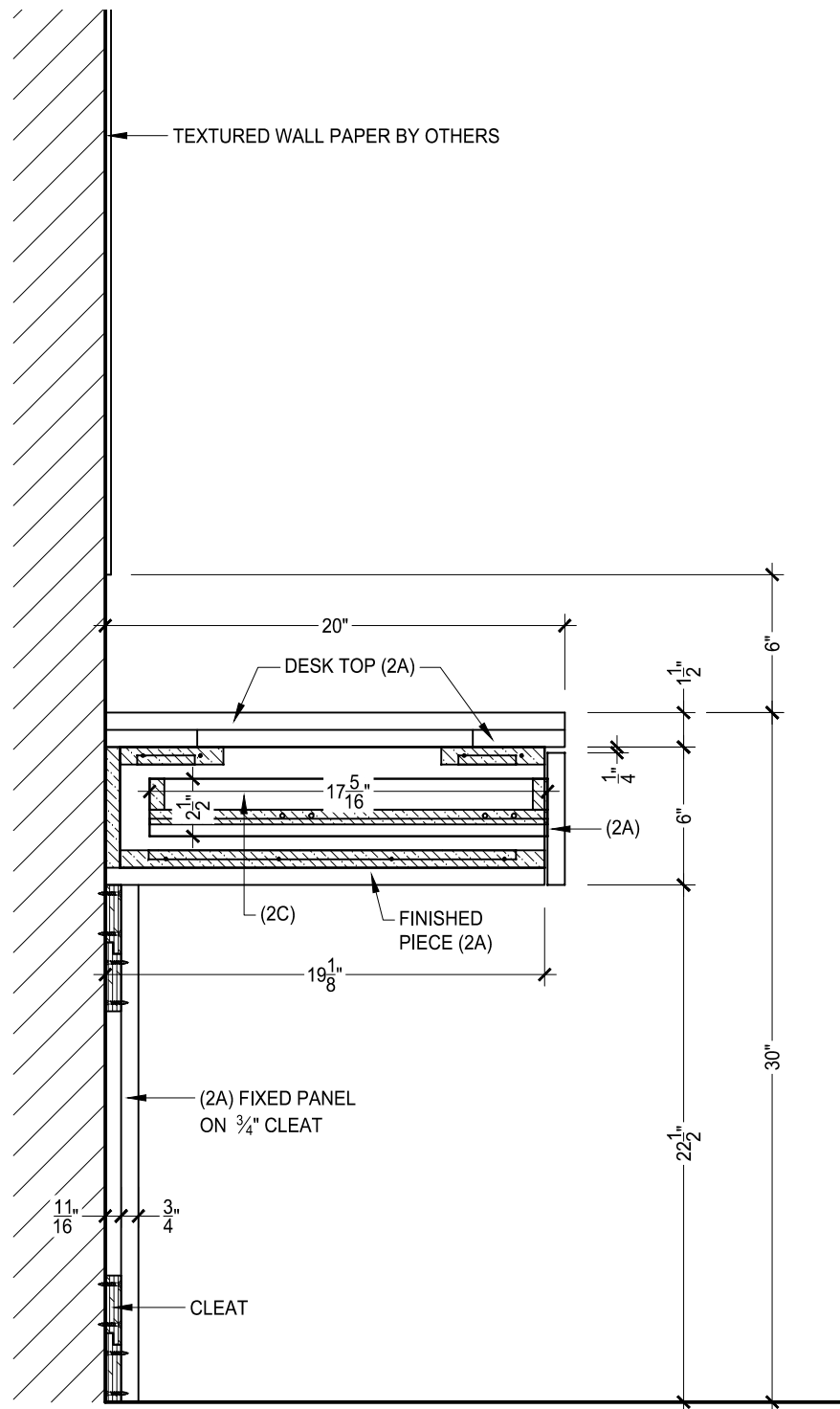
1 SECTION SCALE: 1-1/2" = 1'-0"
