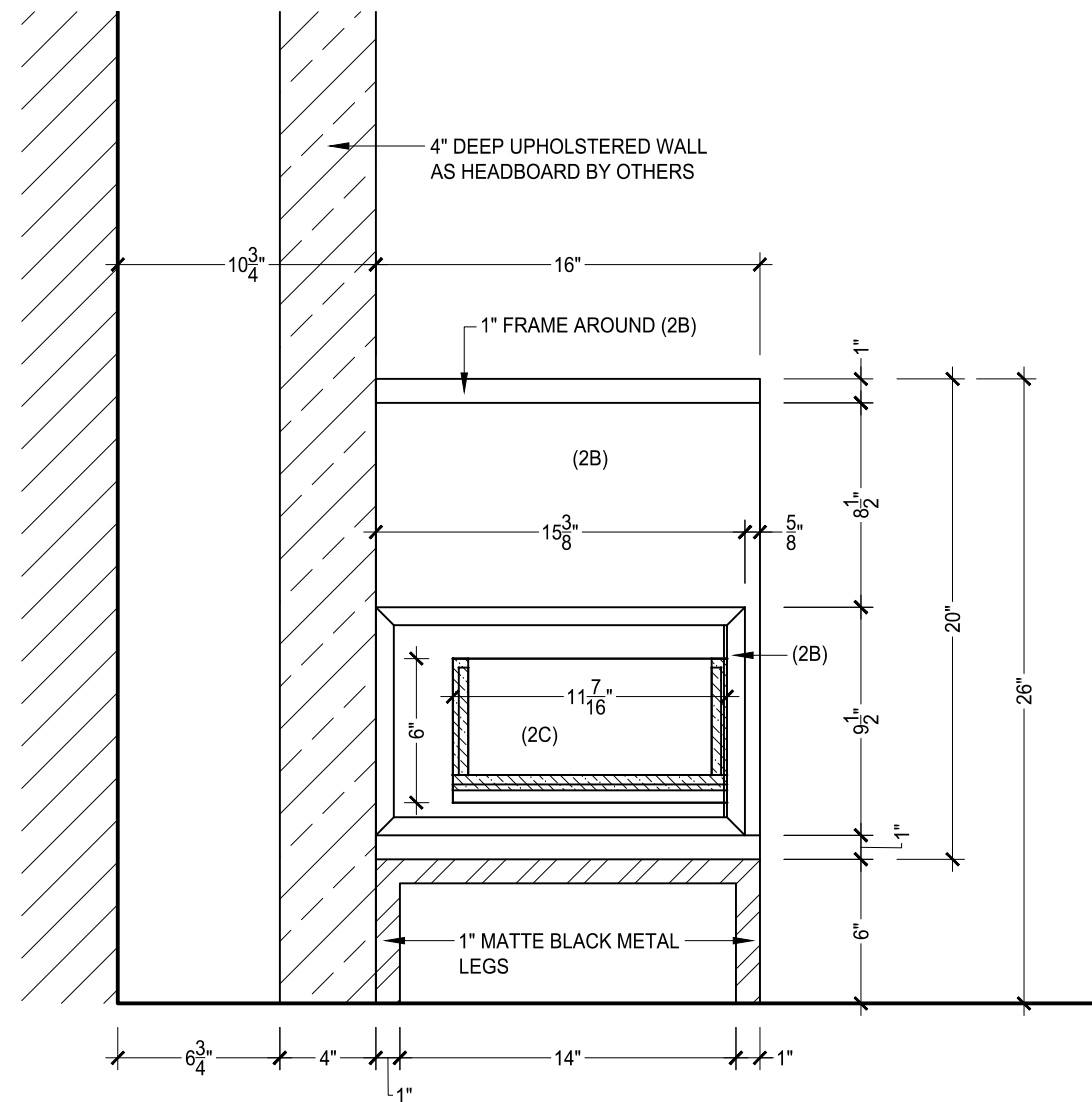
2 SECTION SCALE: 1-1/2" = 1'-0"
