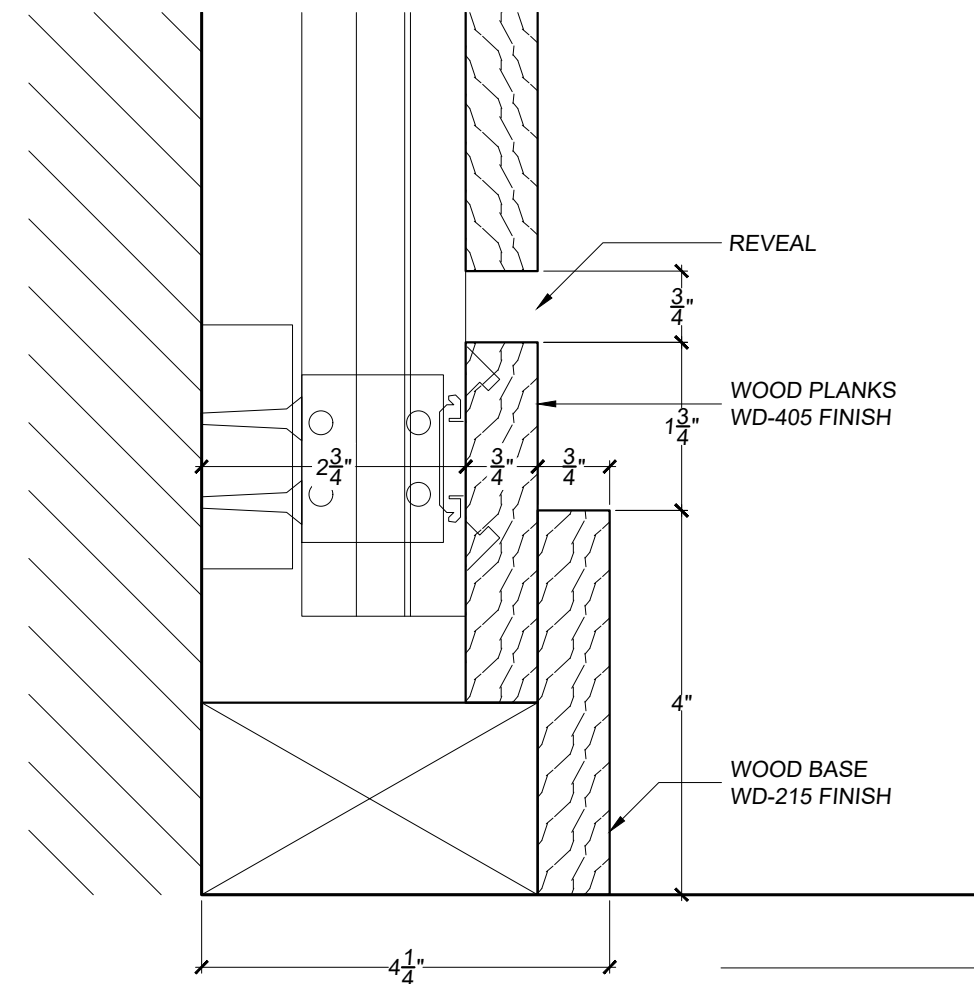
02 2D DETAIL SCALE: 6" - 1'-0" REF.: 11/A802
