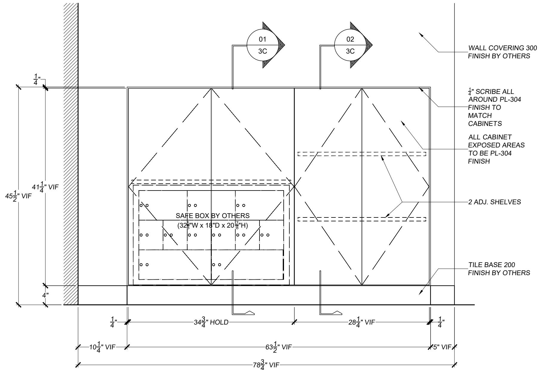
01 3A ELEVATION SCALE: 1" = 1'-0" REF.: 2/A802
