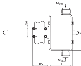
BMV + TTB
