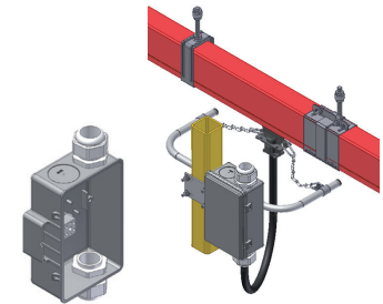
BMV35 + TTB35-4
