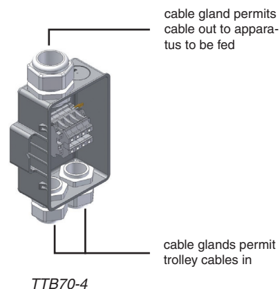
TTB70-4
