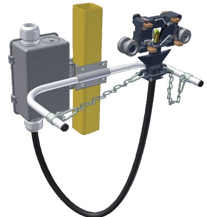
CL4-40/BMV/TTB
