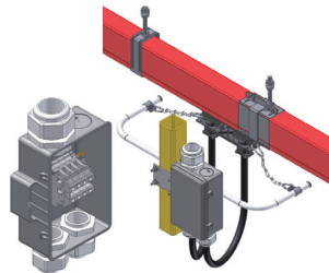
BMV70 + TTB70-4
