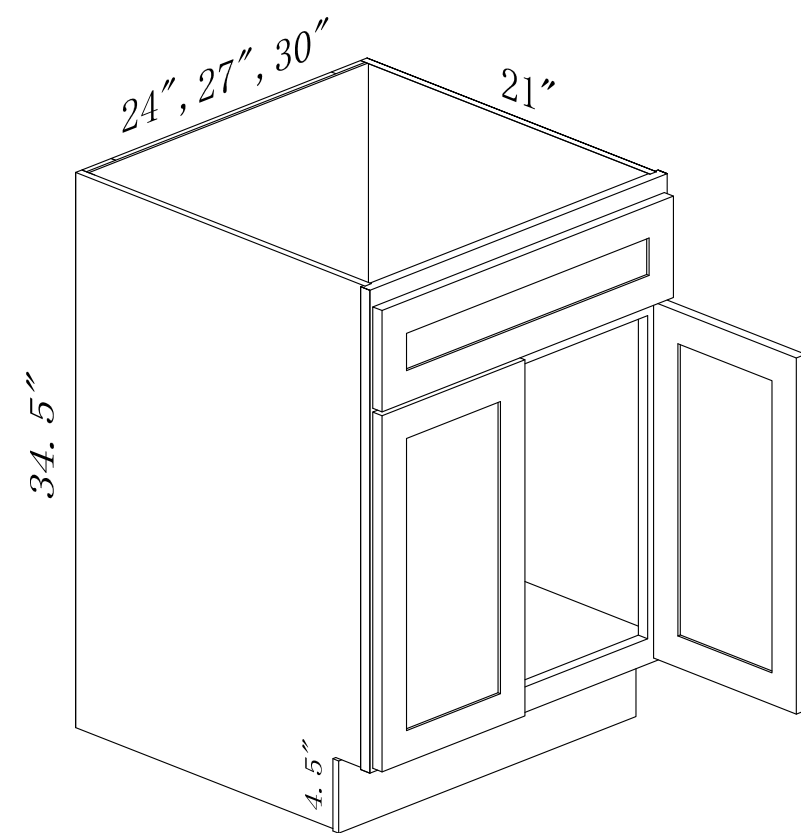
VS24, VS27, VS30
