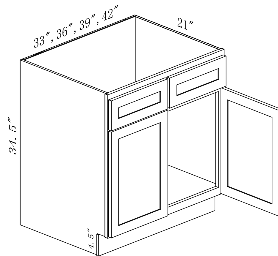
VS33, VS36, VS39, VS42
