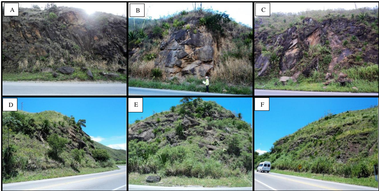
Figura 10 - Talude TI. Vista do trecho mais crítico (A). Talude TC. Vista do trecho mais crítico (B - Talude TB-3. Vista do trecho mais crítico (C) - Talude TB-1 com destaque para a foliação subparalela ao talude (D). TB-2 (E) com destaque para bloco caído. Talude TA-4. Vista lateral com afloramentos altos inacessíveis (F).
