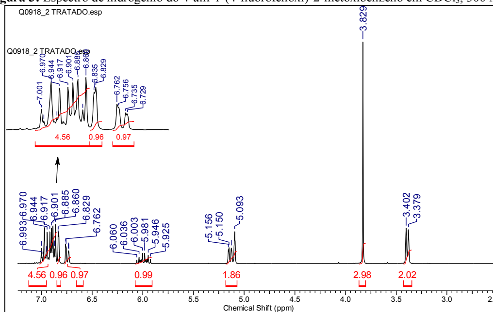
Figura 3: Espectro de hidrogênio do 4-alil-1-(4-fluorofenoxi)-2-metoxibenzeno em \text{CDCl}_3 , 300 MHz
