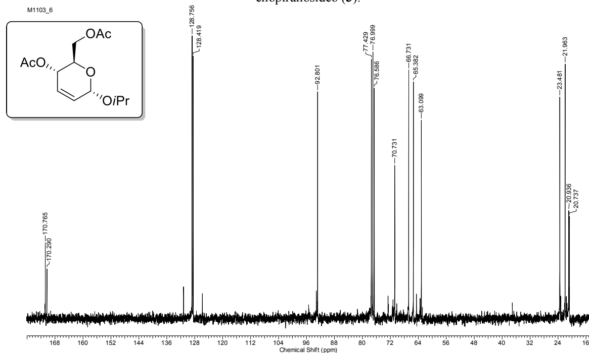
Figura 3: Espectro de RMN ^{13}\text{C} (75 MHz, \text{CDCl}_3 ) do iso -propil 4,6-di- O -acetil-2,3-didesoxi- \alpha -D- eritro -hex-2-enopiranosídeo ( 3 ).
