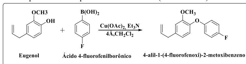
Figura 2: Esquema reacional para a síntese do 4-alil-1-(4-fluorofenoxi)-2-metoxibenzeno.
