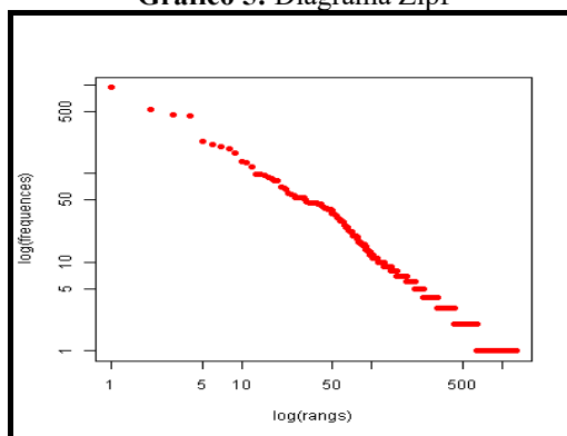
Gráfico 5: Diagrama Zipf
