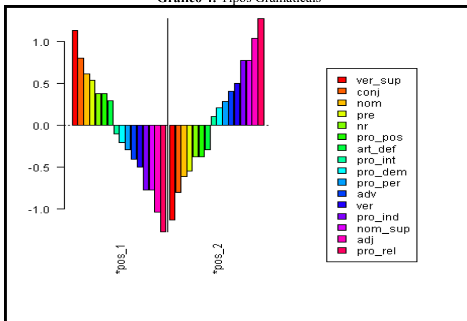
Gráfico 4: Tipos Gramaticais
