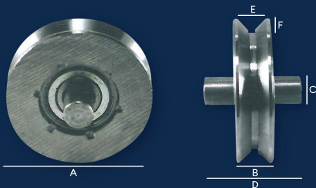
ROLDANA PARA PORTÃO - CAVA V (CANTONEIRA) - SEM SUPORTE
