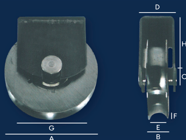
ROLDANA PARA PORTÃO - CAVA U - FERRO 1/2 Ø - COM SUPORTE
