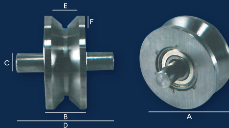
ROLDANA DUPLA / 02 ROLAMENTOS - CAVA V (CANTONEIRA) - SEM SUPORTE
