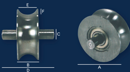
ROLDANA DUPLA / 02 ROLAMENTOS - CAVA U - TUBO 1/2 Ø - SEM SUPORTE
