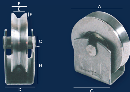
ROLDANA PARA PORTÃO - CAVA V (CANTONEIRA) - COM SUPORTE
