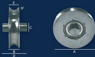
ROLDANA PARA PORTÃO - CAVA U - FERRO 1/2"Ø - SEM SUPORTE
