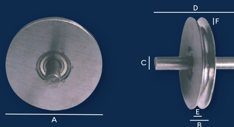
ROLDANA PARA PORTA DE CONTRAPESO
