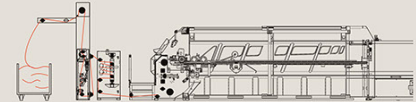
Salıncak Ortalayıcılı Giriş / Swing Type Fabric Centering
