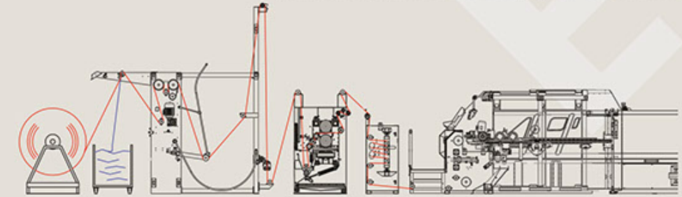
Parmak Tutuculu Giriş - Non Stop J-Box / Finger Type Cloth Guider - Non Stop J-Box
