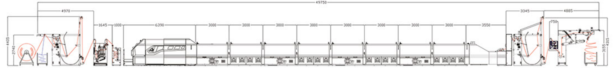
Denim ve Üst Giyim Dokuma Kumaşlar için Non-Stop Giriş Çıkışı Temel Ram Hattı / Main Stenter Line for Denim and Outwear Woven Fabrics With Non-Stop Entrance and Exit
