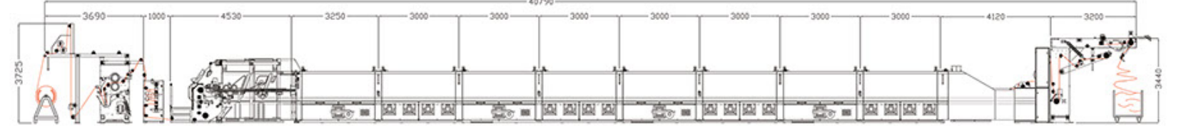
Dokuma Kumaşlar için Tek Fularlı Temel Ram Hattı / Main Stenter Line For Woven Fabrics With Single Padder
