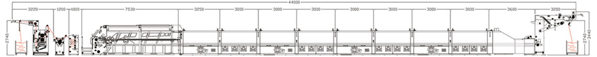
Döşemelik Dokuma Kumaşlar için Sırt Apre Üniteli Temel Ram Hattı / Main Stenter Line For Upholstery Woven Fabrics With Backcoating Unit
