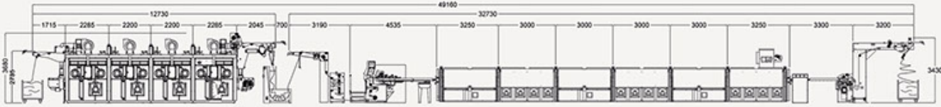
Kumaş Kurutma ve Terbiye Hattı / Fabric Drying and Finishing Line
