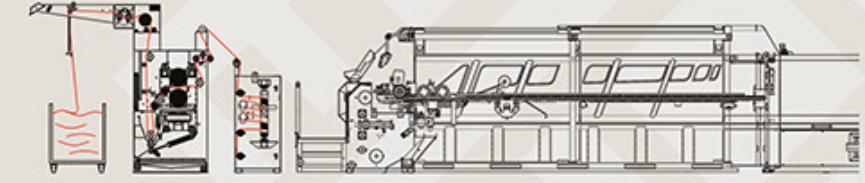
Çıtalı Açılıcılı Giriş - Tek Fular / Web Guiding System - Single Padder
