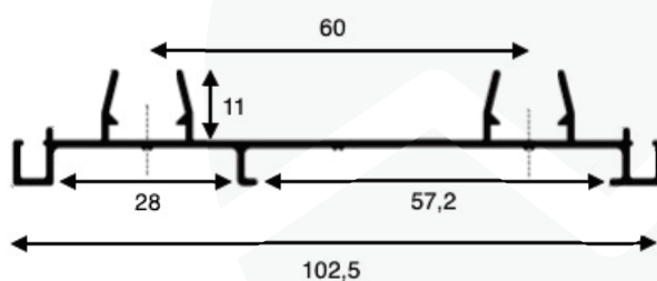
EXM-36 - Peso 0,656 kg/m
