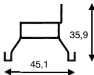
EXE-381 - Peso 0,256 kg/m
