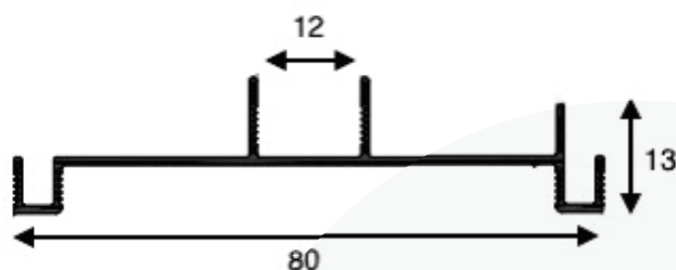
EXE-1205 - 0,272 kg/m
