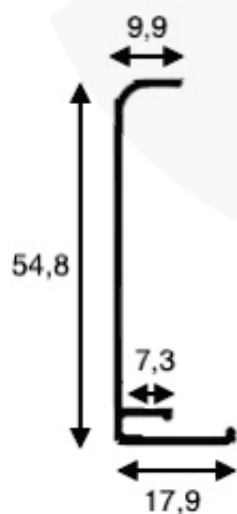
MAG -2 - 0,237 kg/m
