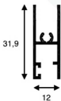
EXE-1219 - Peso 0,211 kg/m
