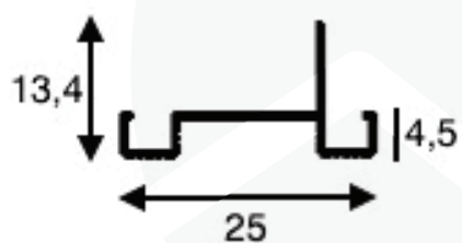
EXE-169 - Peso 0,105 kg/m
