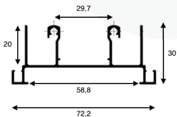
EXM-66 - Peso 0,769 kg/m
