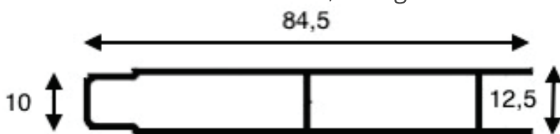
ELB-004 - Peso 0,619 kg/m
