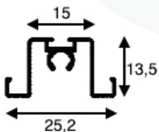
EXE-170 - Peso 0,174 kg/m
