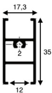
EXF-10 - Peso 0,283 kg/m
