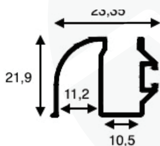
EXB-502 - Peso 0,252 kg/m
