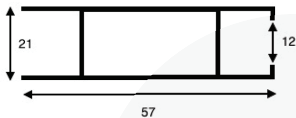
ESU-238 - 0,403 kg/m
