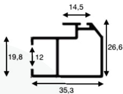
EXF-03 - Peso 0,323 kg/m
