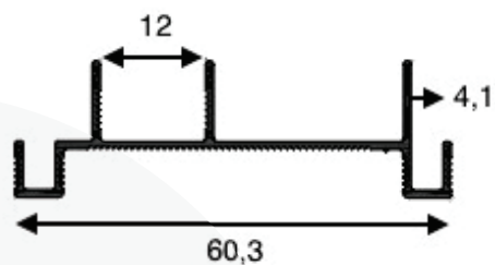
EXE-1208 - Peso 0,230 kg/m
