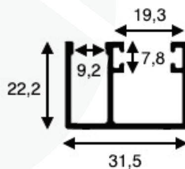
MAG -3 - Peso 0,305 kg/m
