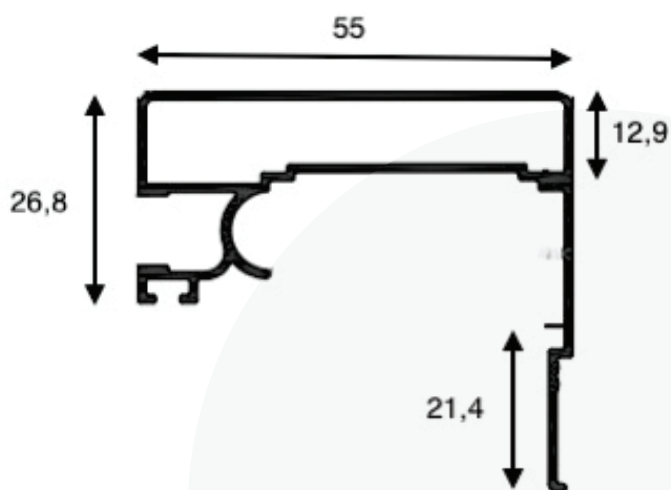
MAG -1 - Peso 0,574 kg/m
