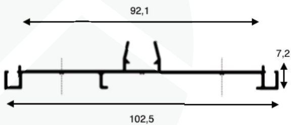
EXM-35 - Peso 0,567 kg/m
