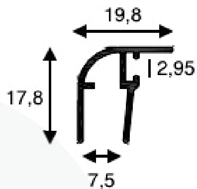
EXB-507 - 0,159 kg/m
