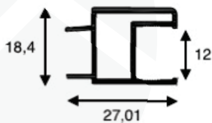
EXE-1218 - Peso 0,209 kg/m
