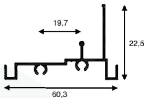
EXE-1212 - Peso 0,289 kg/m
