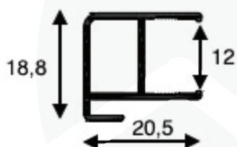
EXE-1213 - Peso 0,167 kg/m
