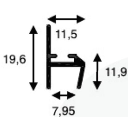
EXB-506 - Peso 0,133 kg/m
