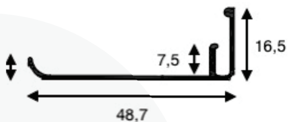
EXB-501 - Peso 0,207 kg/m
