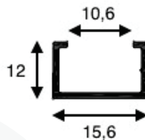
EXE-191- Peso 0,105 kg/m
