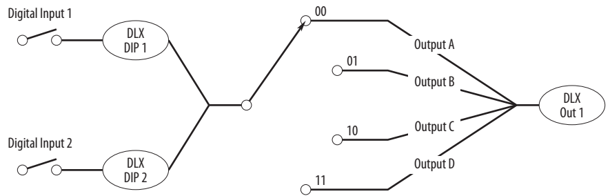
Figura 92 – Mapa lógico del interruptor selector de dos entradas y cuatro posiciones
