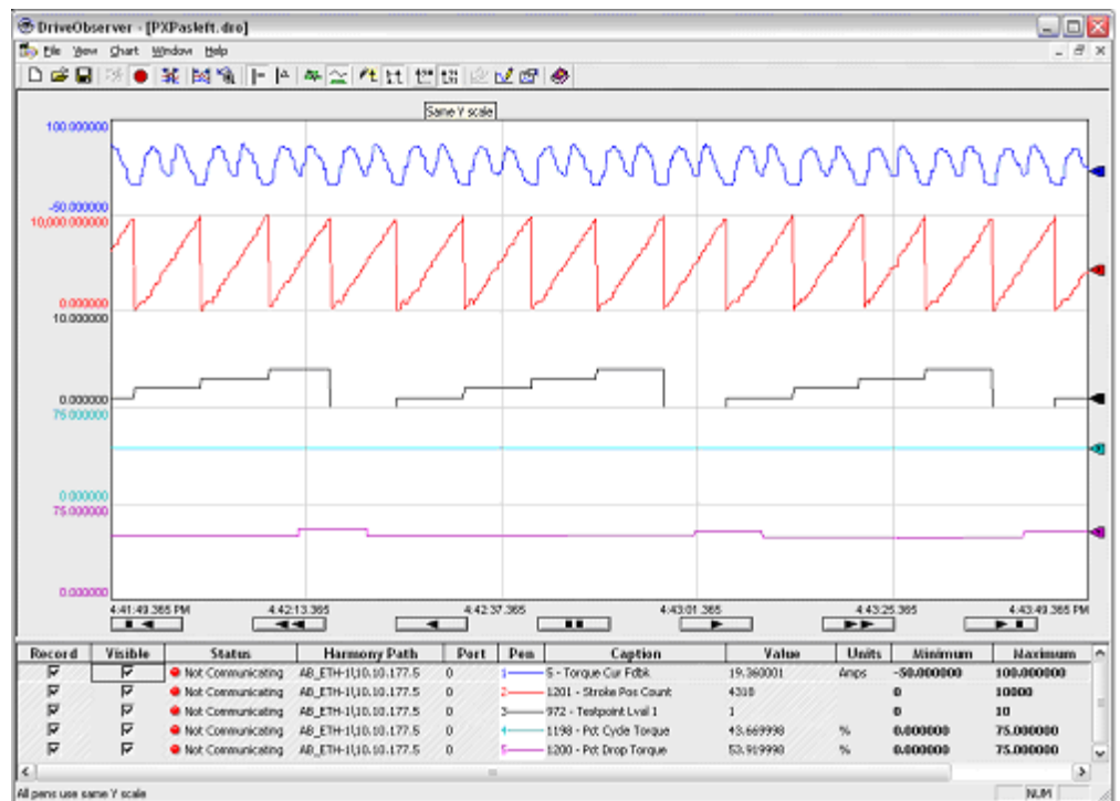
Figura 80 – Ajustes del DriveObserver
