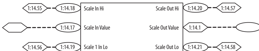
Figura 93 – Vista de bloques a escala en nivel alto
