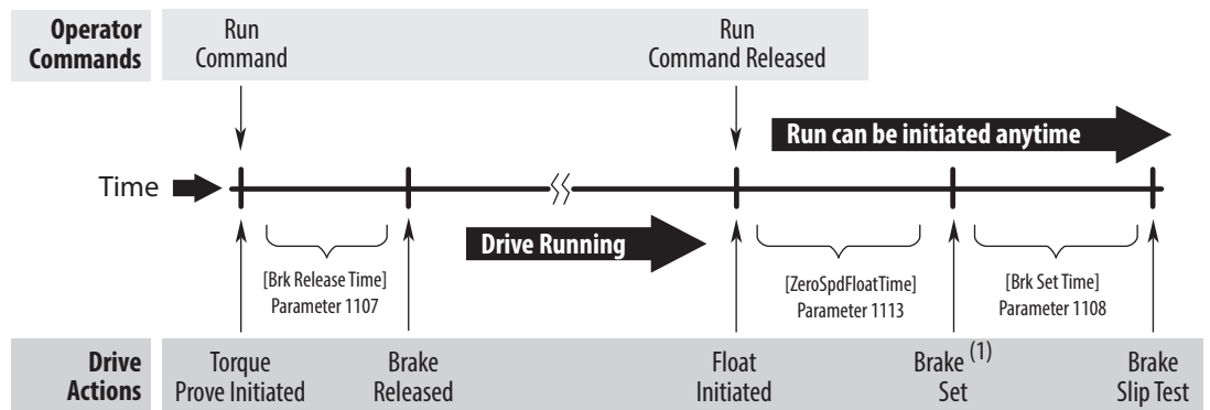
Figura 79 – Diagrama de flujo de prueba de par
