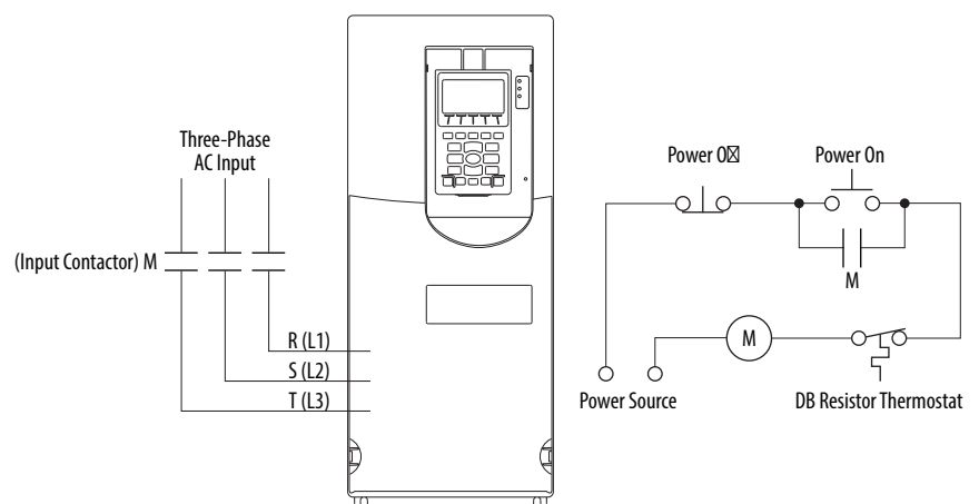
Figura 4 – Circuitos de resistencia externa de freno
