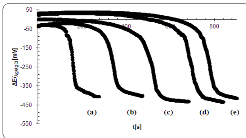
Curvas de titulación de \Delta E/ER=f(t) para cada ensayo de alícuotas de HCl, a) 100 \mu\text{L} , b) 200 \mu\text{L} , c) 300 \mu\text{L} , d) 400 \mu\text{L} y e) 500 \mu\text{L} por microtitulación coulombimétrica a corriente impuesta
