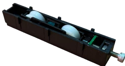
PL4600-150D CARRETILLA 150 KG
