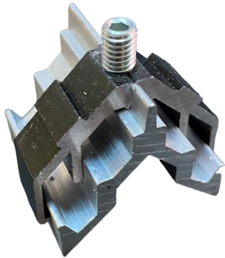
ES1311NA ESCUADRA VENTANA
