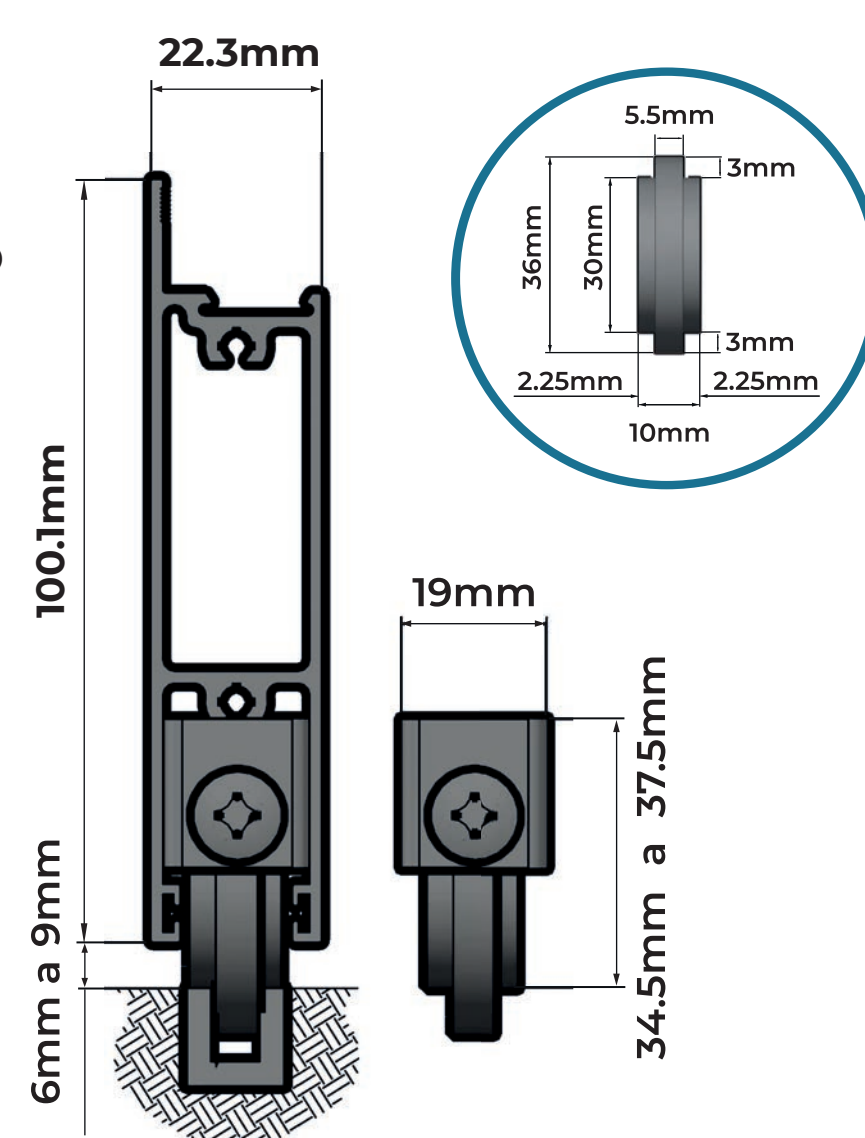
ROLDANA SUPREMA CANALETA ESCOVA P/ DENTRO
