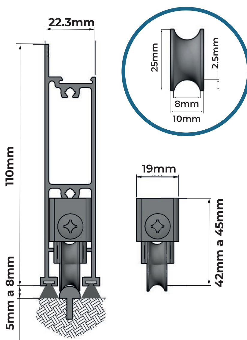
ROLDANA SUPREMA MEIA-CANA ESCOVA P/ BAIXO
