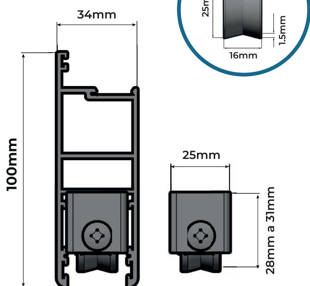
ROLDANA EUROSHOW CONVENCIONAL
