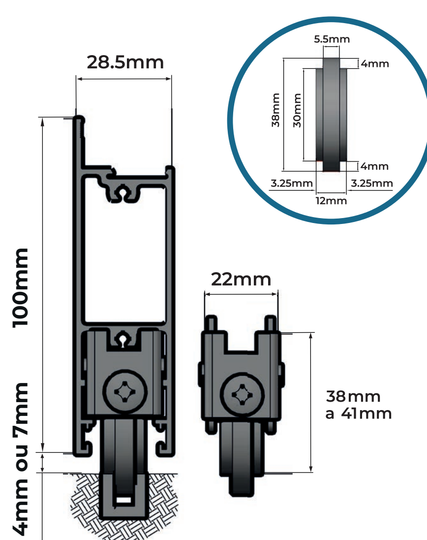
ROLDANA GOLD CANALETA ESCOVA P/ DENTRO
