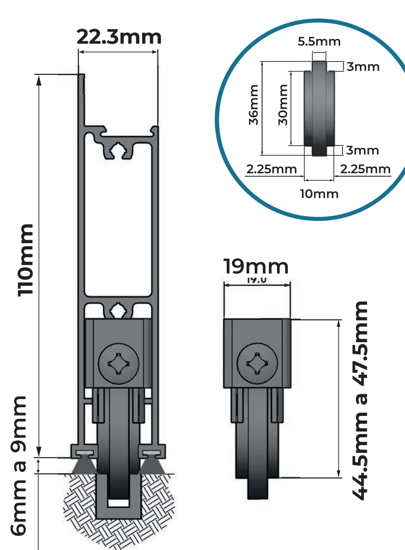
ROLDANA SUPREMA CANALETA ESCOVA P/ BAIXO
