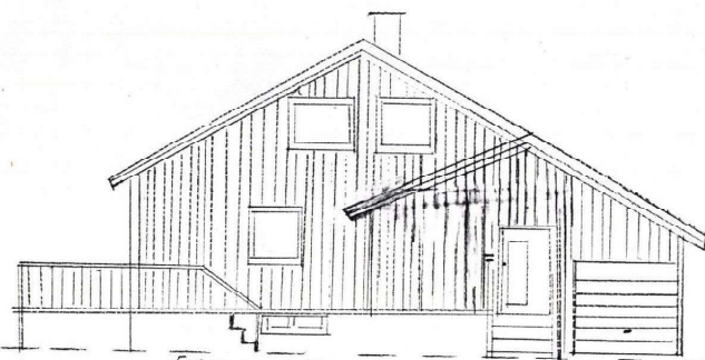
FASADE SYD
