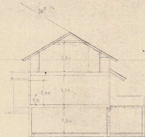
SNITT
