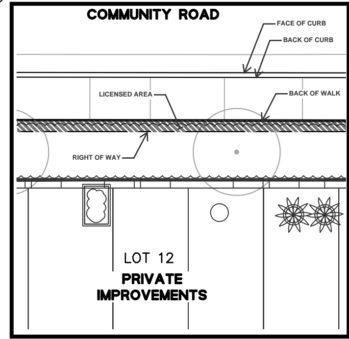
ENLARGEMENT SCALE 1:10
