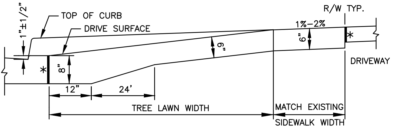
SECTION A-A
