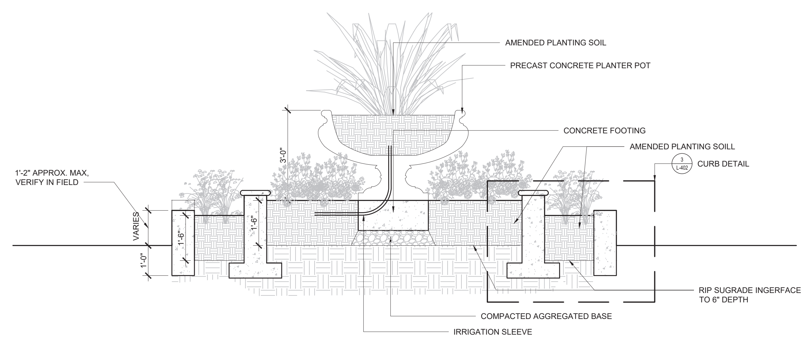
2 LA CUESTA MEDIAN SECTION SCALE: 1/2" = 1'-0"
