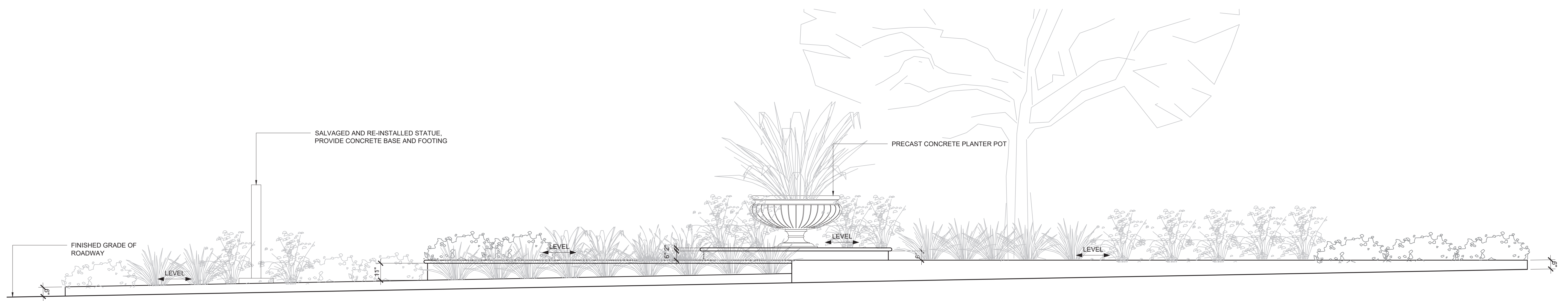
1 LA CUESTA MEDIAN ELEVATION SCALE: 3/8" = 1'-0"
