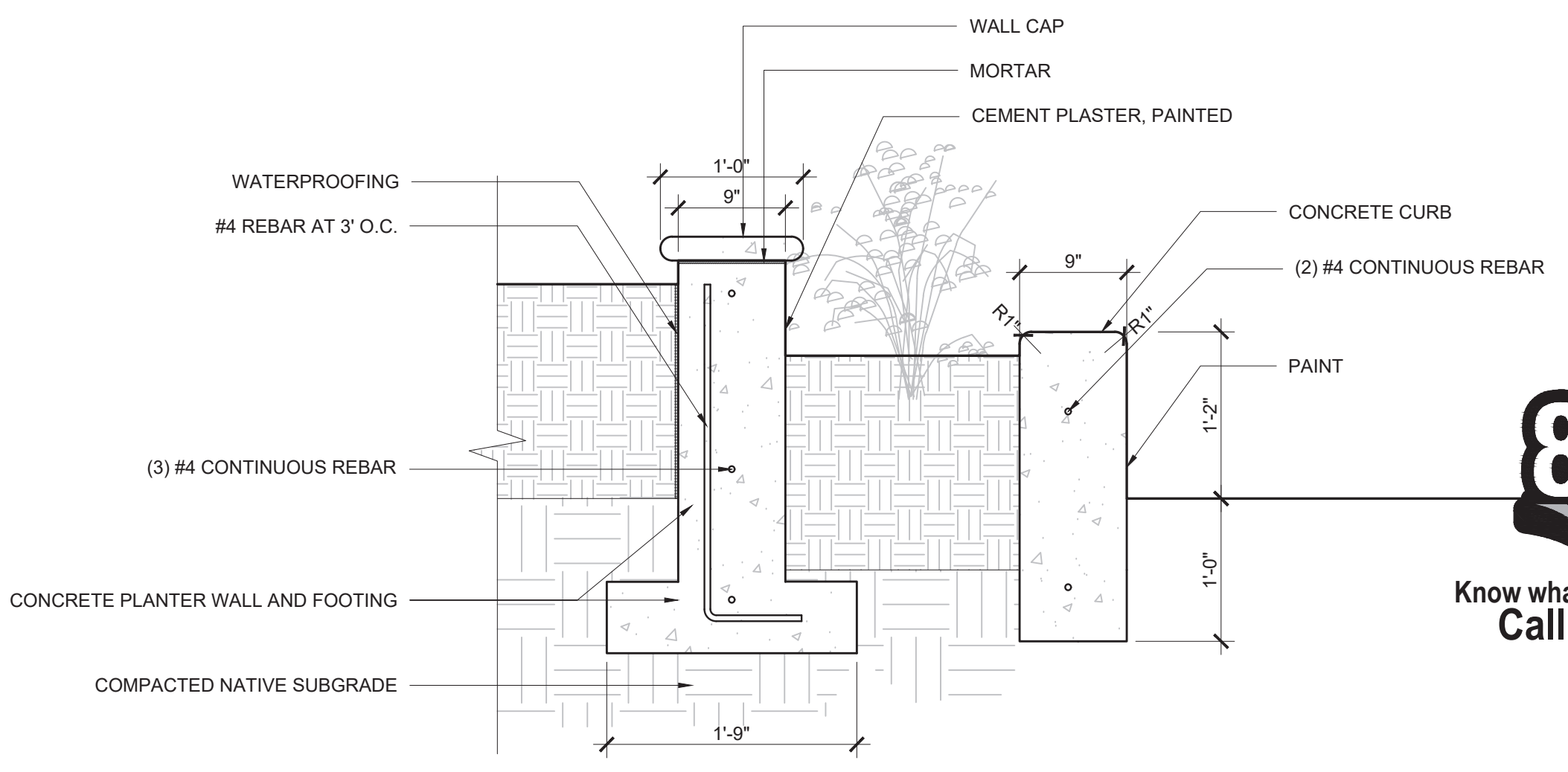
3 LA CUESTA MEDIAN CURB DETAILS SCALE: 1" = 1'-0"
