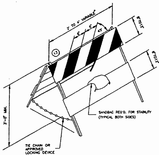
BARRICADE TYPE I
