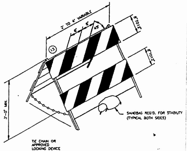
BARRICADE TYPE II
